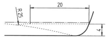
SEITENANSICHT BODENNOCKE M 2:1
